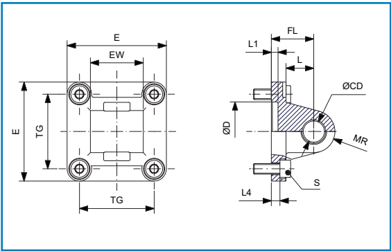
Cerniera maschio MP4 Male hinge MP4
